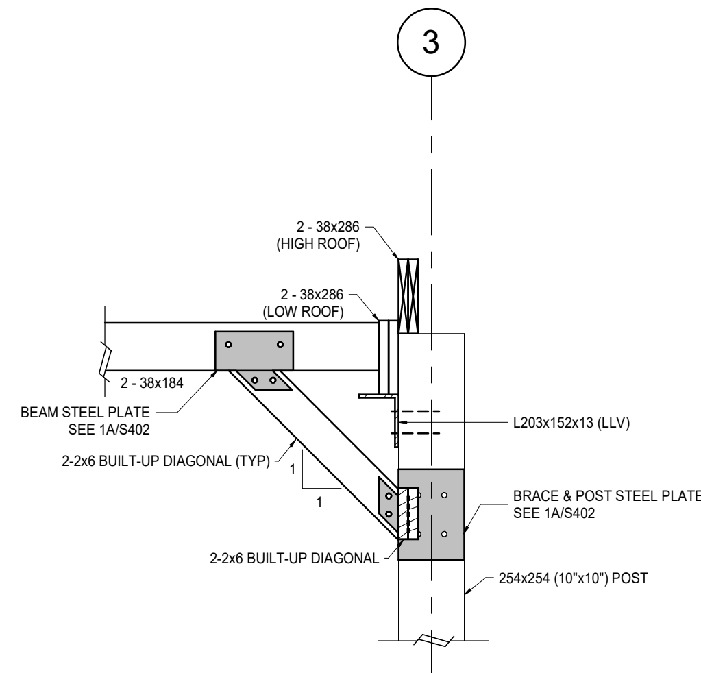
1B SECTION S402 1 : 20
