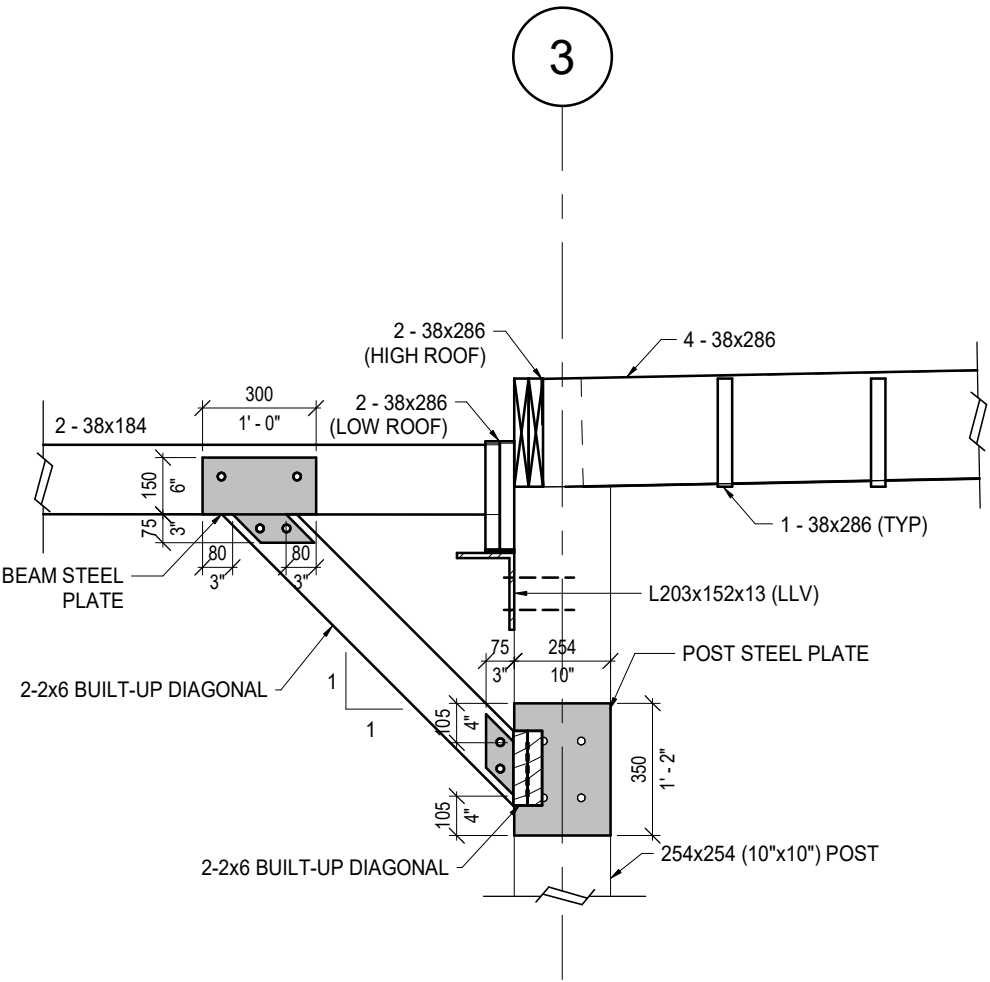
1A SECTION S402 1 : 20
