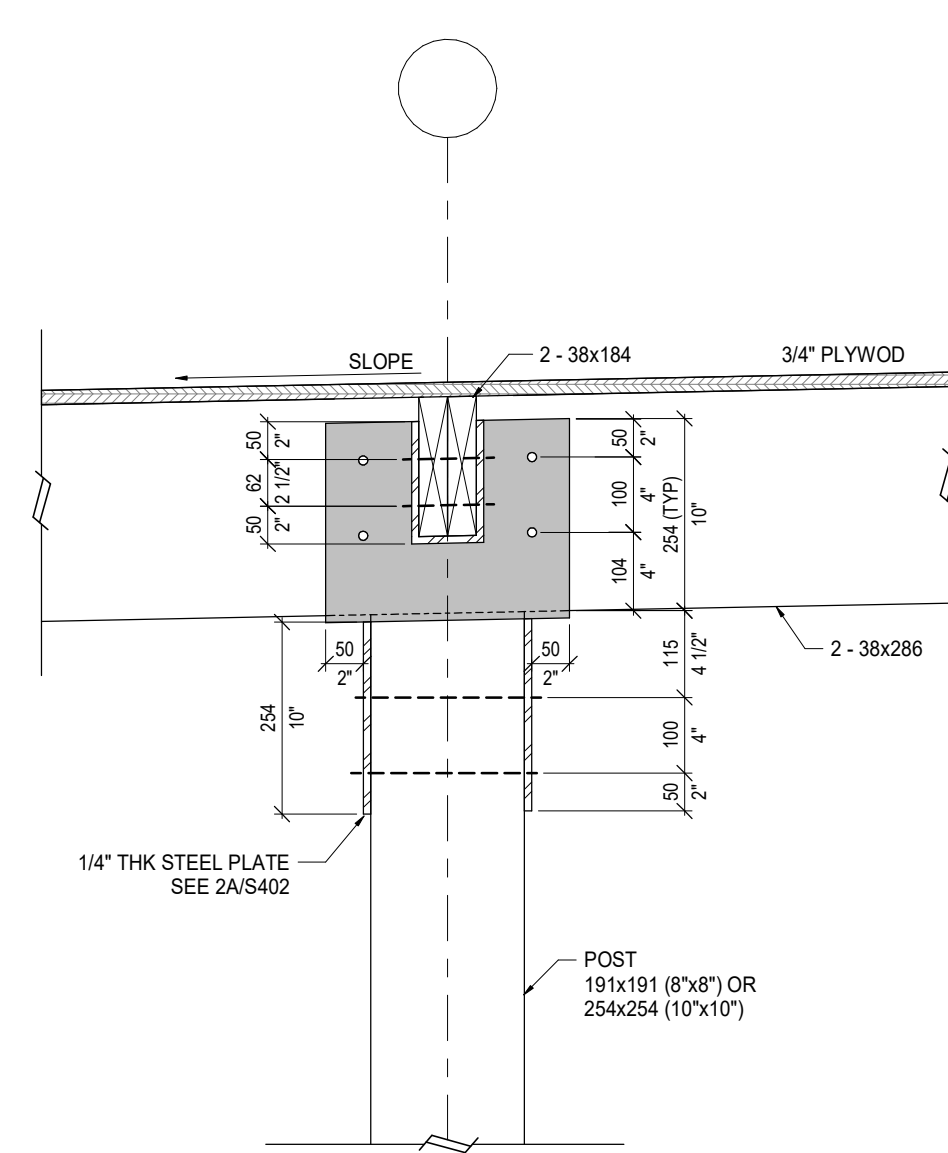
2 SECTION S402 1 : 10
