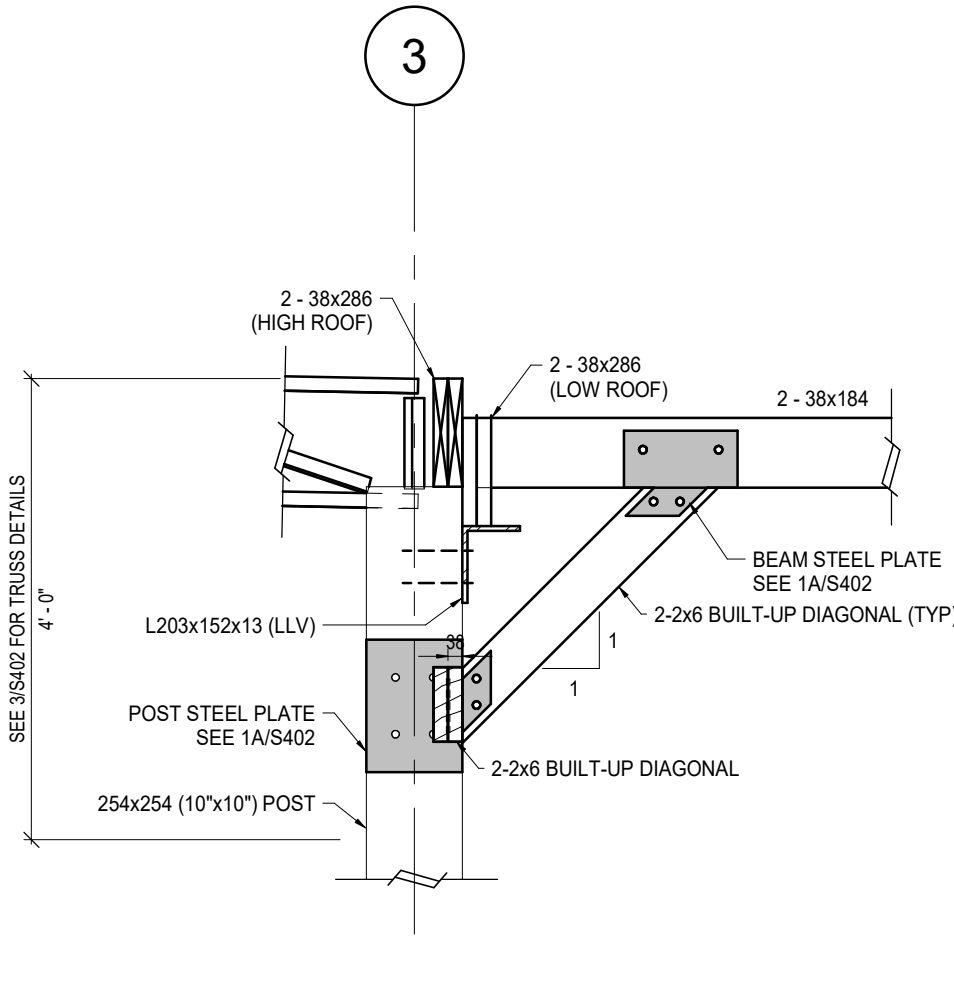
1C SECTION S402 1 : 20
